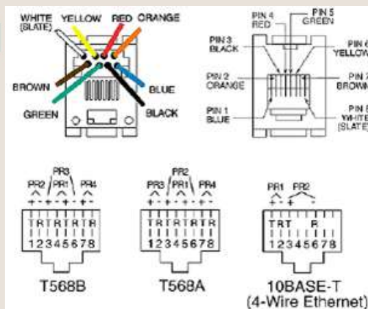
Figura 3 - Pinagens para RJ45 fêmea
