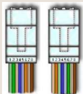
Figura 1 - Padrões 568A e 568B
