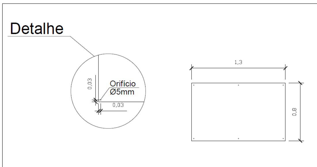
Figura 1: Croqui de furação (orifícios) da placa do tipo "Aviso de Alerta"
