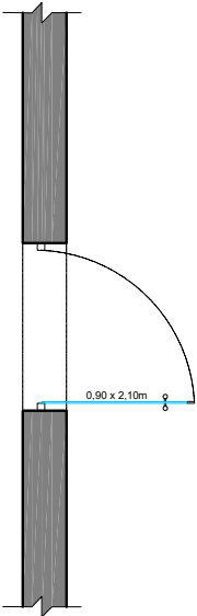
PLANTA BAIXA PORTA DE VIDRO ESC 1/50
