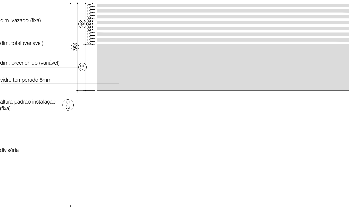
DETALHE PADRÃO - VISTA DIVISÓRIA + VIDRO ESC.: 1/20
