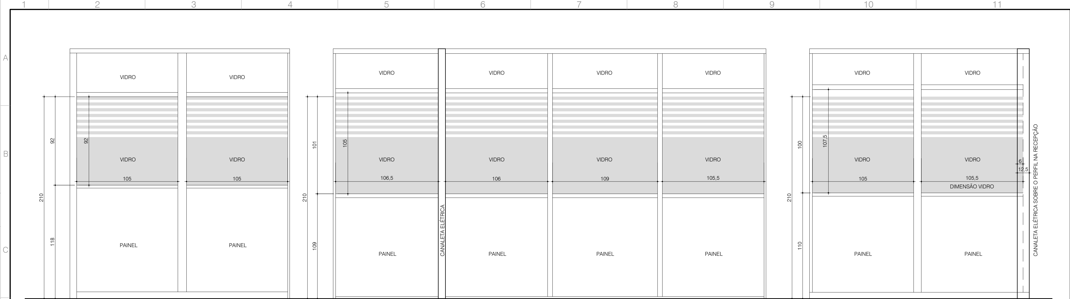
DETALHE 3 - VISTA 3 ESC.: 1/20
