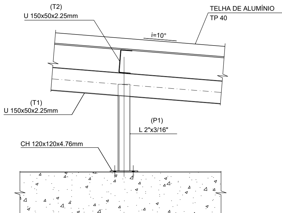
DETALHE APOIO DAS TERÇAS
