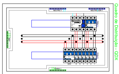
15 EXEMPLO DE EXECUÇÃO DE QUADRO DE DISTRIBUIÇÃO
