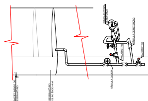
DETALHE DA BOMBA E FUNCIONAMENTO
