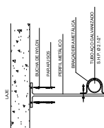
TUBULAÇÃO DE S.H.P. SUSPENSÃO
