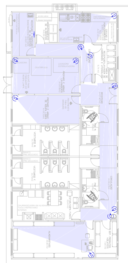
PLANTA BAIXA - P17 - SERVIÇOS
