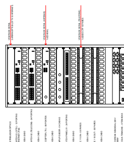
RACK P20 (20U) ATIVO / PASSIVO
