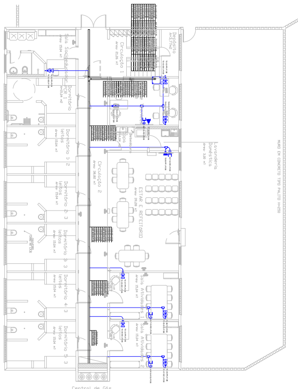
PLANTA EMBA TERREO - P1/98 - INTERNAÇÃO FASE FINAL (ICPAE)
