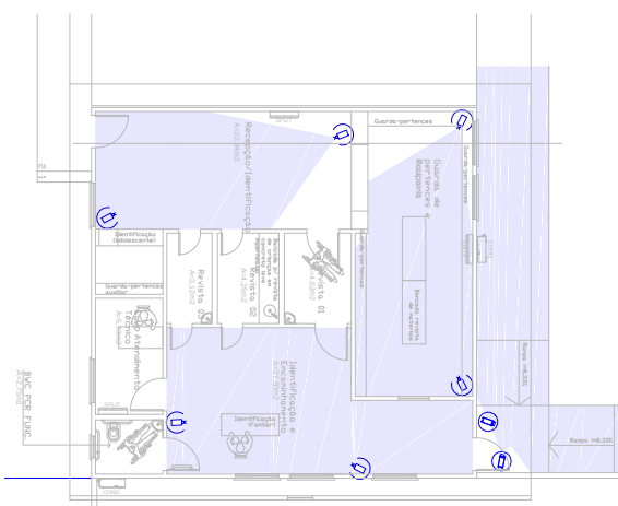
PLANTA BAIXA - P19 - REVISTA
