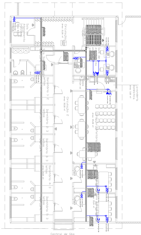
PLANTA BAIXA SUPERIOR - P158 - INTERNAÇÃO FASE FINAL (ICPAE)
