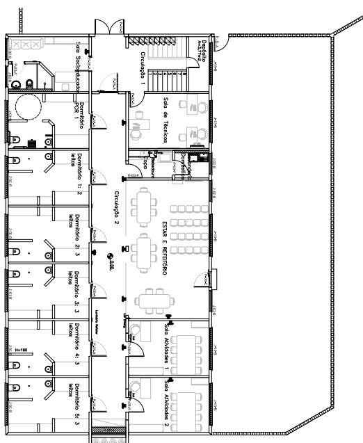
PLANTA BAIXA - SUPERIOR Escala: 1/100
