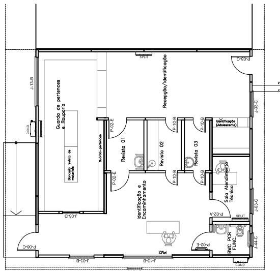
PLANTA BAIXA ESCALA 1:100 P19 - REVISTA
