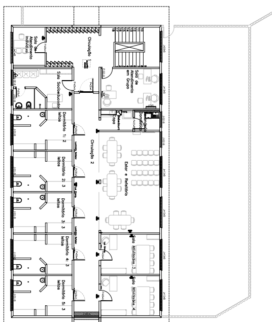
PLANTA BAIXA - SEGUNDO PAVIMENTO Escala: 1/100
