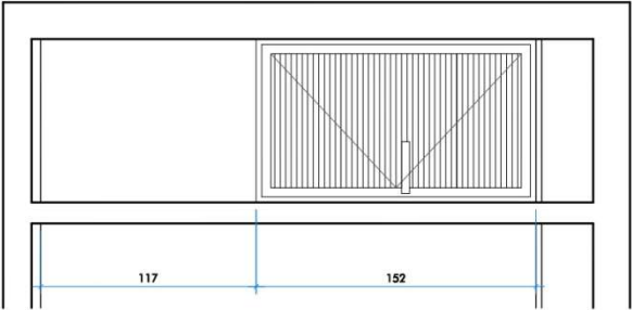
VISTA FRONTAL ESCALA 1:25
