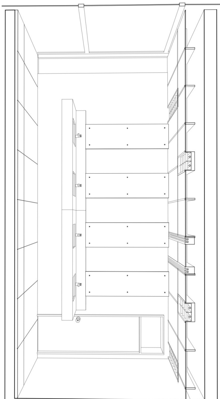
PERSPECTIVA FRONTAL SEM ESCALA
