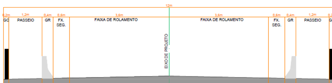
Fig. 4: Seção- tipo exigida
