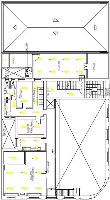
PLANTA BAIXA MEZANINO ESCALA 1:125
