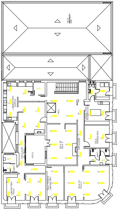
PLANTA BAIXA SEGUNDO PAVIMENTO ESCALA 1:125
