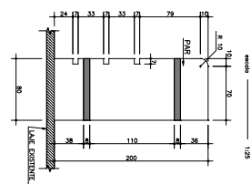
CORTE A-A 12
