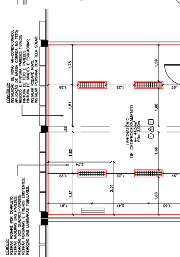
01 A DEMOLIR/ CONSTRUIR LABORATÓRIO DE GEOPROCESSAMENTO - SALA 32
