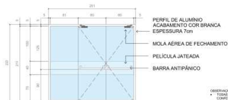
3 DIVISÓRIA B VISTA POSTERIOR
