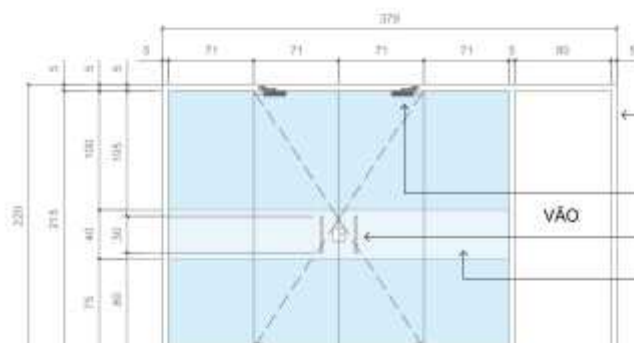
2 DIVISÓRIA A VISTA FRONTAL
