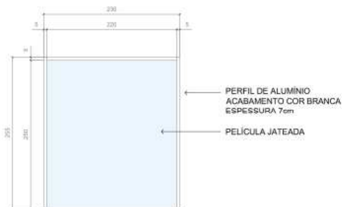
2 DIVISÓRIA E VISTA FRONTAL
