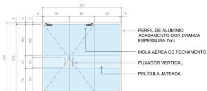
2 DIVISÓRIA B VISTA FRONTAL
