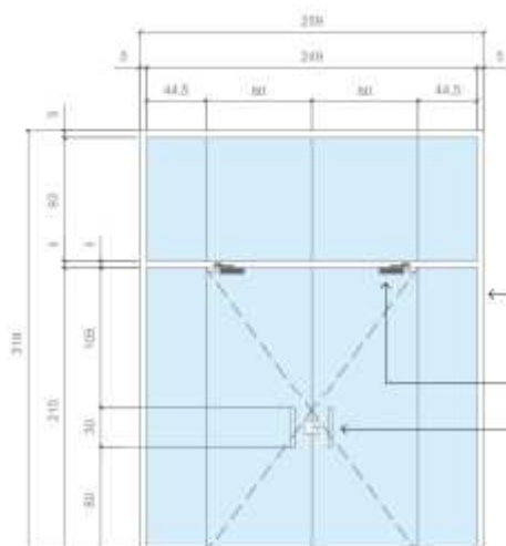
2 DIVISÓRIA C VISTA FRONTAL
