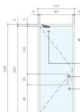
2 DIVISÓRIA G VISTA FRONTAL
