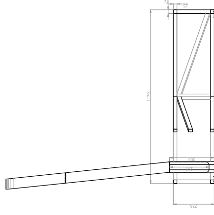
CORTE C1
