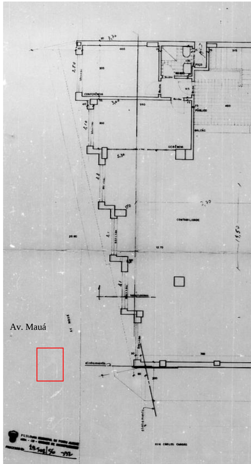
Figura 6 – Planta original do Projeto Arquitetônico (Av. Mauá)
