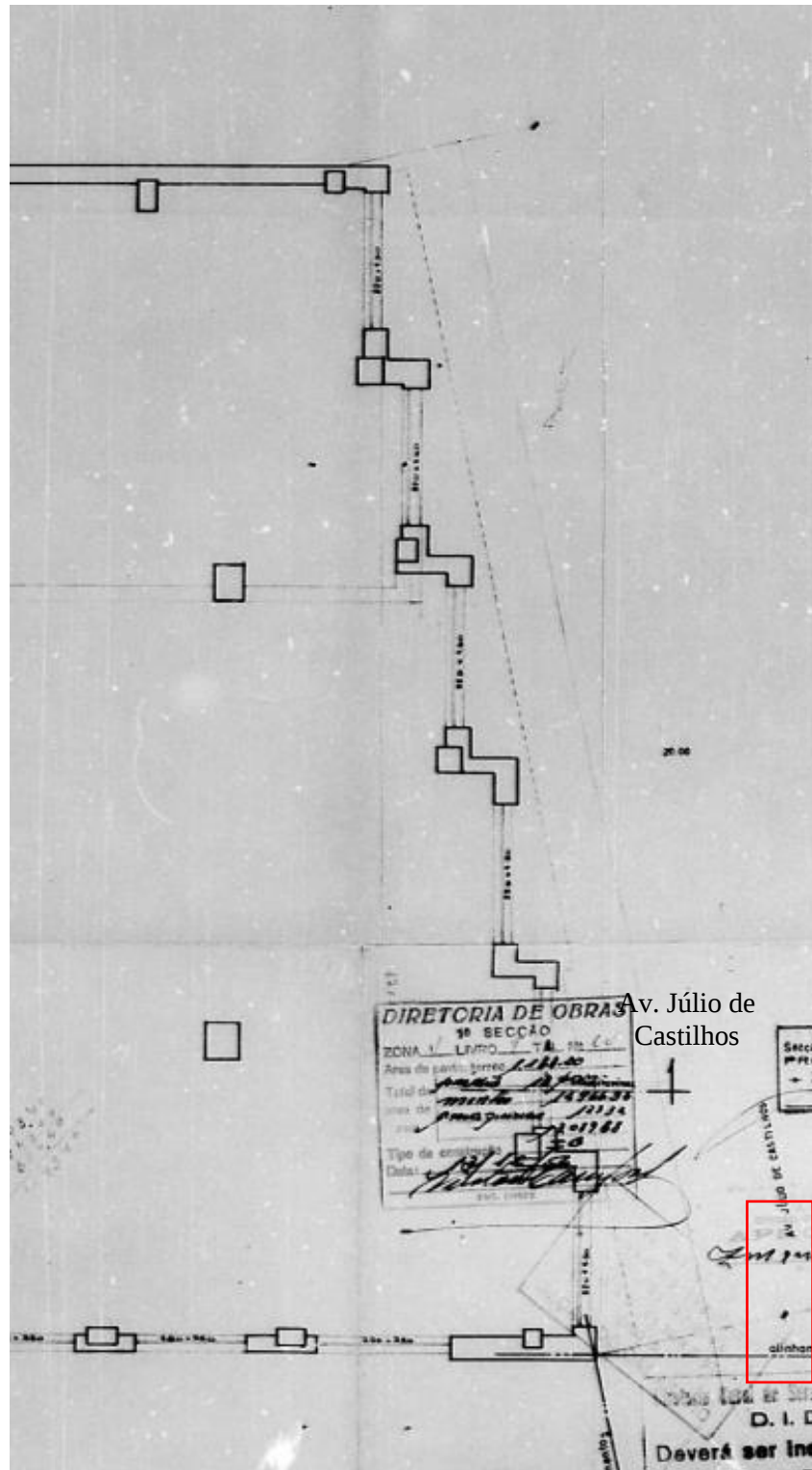
Figura 7– Planta original do Projeto Arquitetônico (Av. Júlio de Castilhos)
