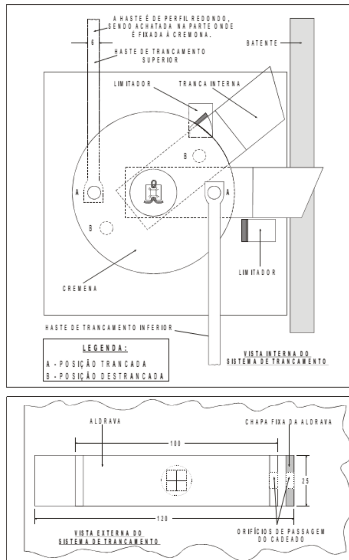
Fig 17 - Vista do sistema de trancamento da porta nas posições trancada e destrancada (medidas em mm)
