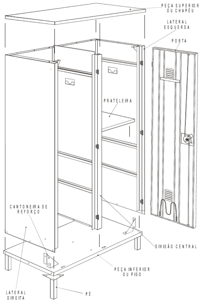
Fig 3 - Vista do armário desmontado
