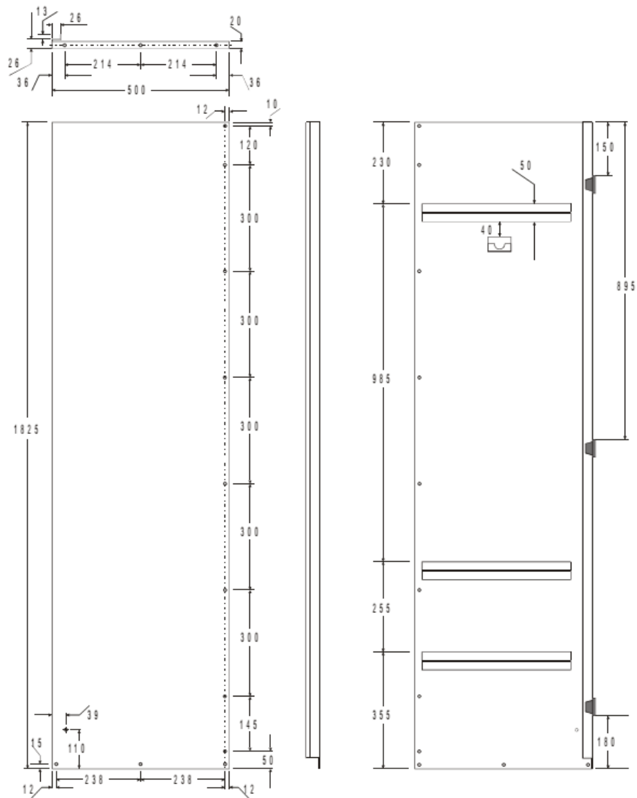
Fig 9 - Vista da lateral esquerda do armário (medidas em mm)
