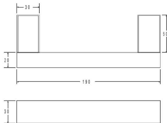
Fig 21 - Porta-cinto (medidas em mm)
