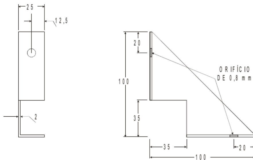
Fig 22 - Cantoneira de reforço (medidas em mm)
