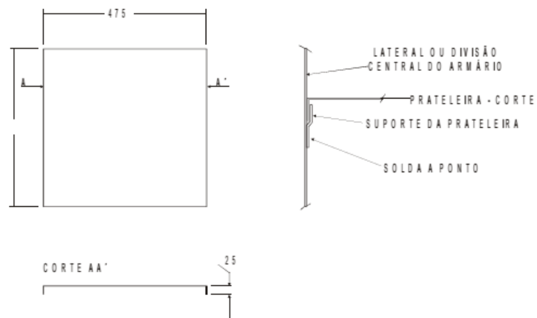
Fig 19 - Vista da prateleira e detalhe de fixação da mesma (medidas em mm)
