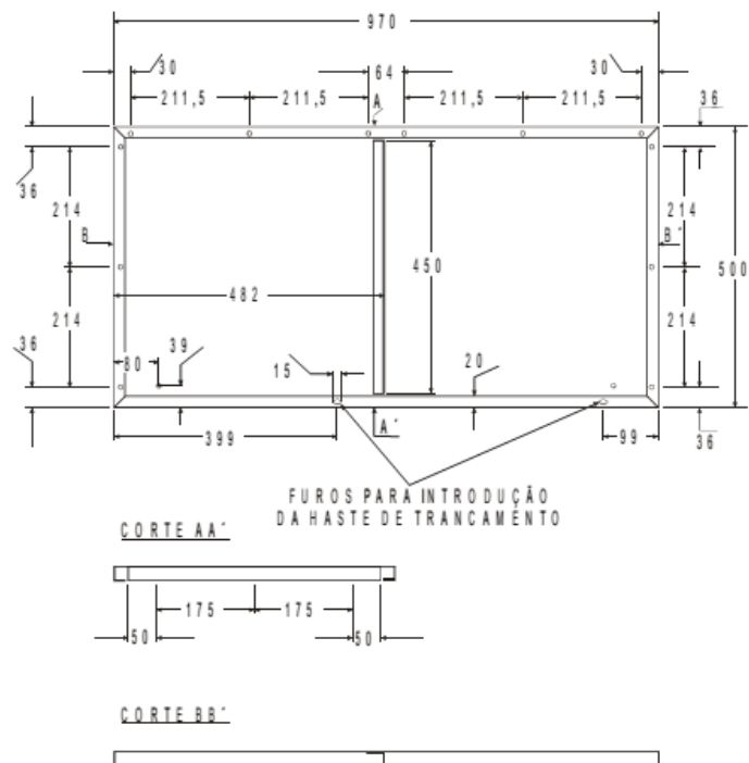
Fig 7 - Vista da parte inferior do chapéu do armário (medidas em mm)
