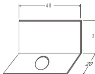
Fig 13 - Guia da haste de trancamento da porta (medidas em mm)
