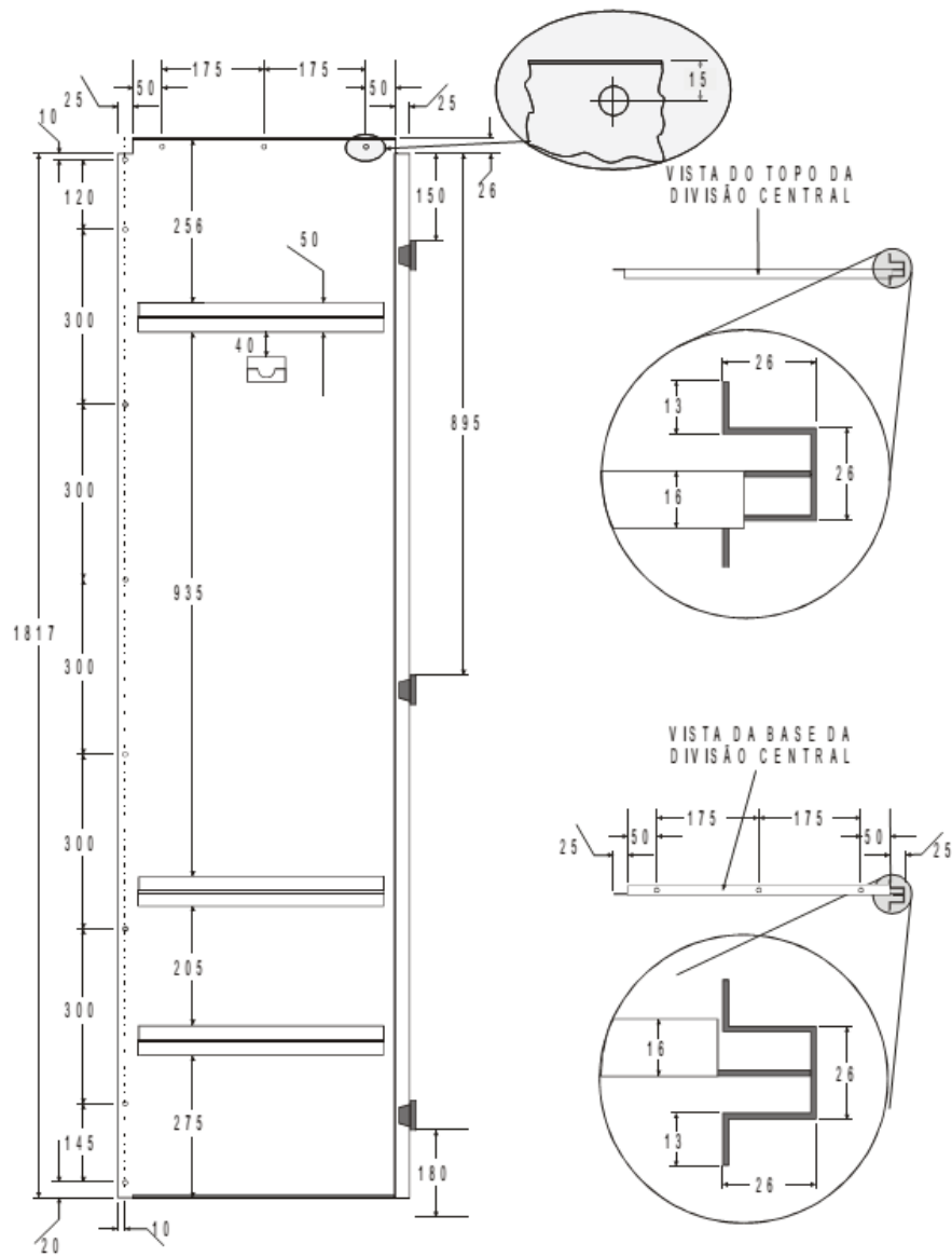
Fig 10 - Vista da divisão central do armário (medidas em mm)
