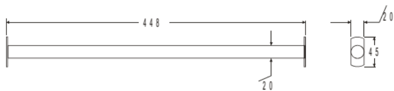
Fig 20 - Cabideiro (medidas em mm)
