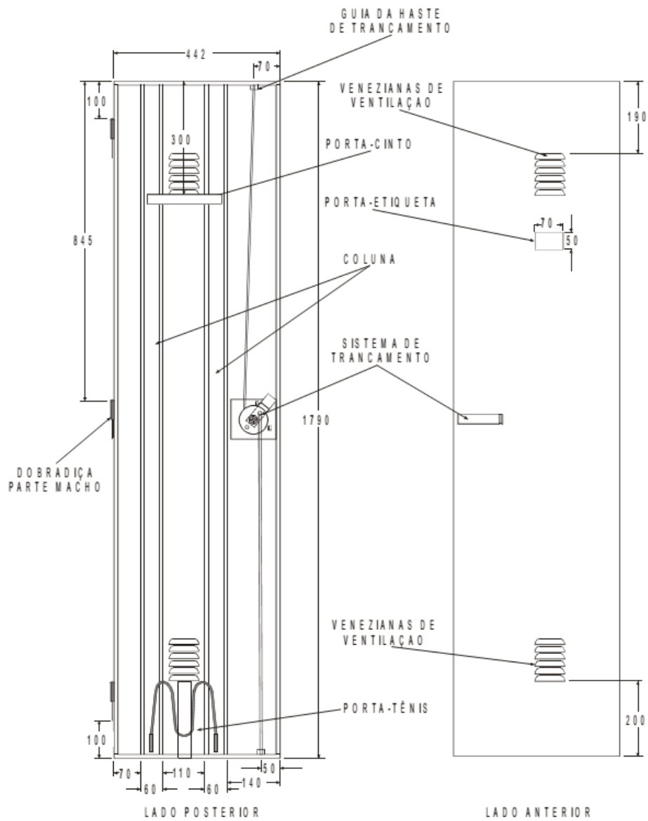
Fig 11 - Porta do armário (medidas em mm)
