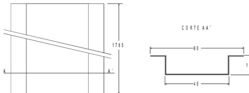
Fig 12 - Coluna da porta (medidas em mm)
