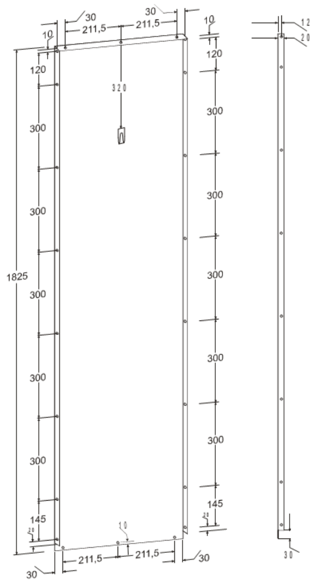
Fig 18 - Vista do lado traseiro esquerdo do armário (medidas em mm)
