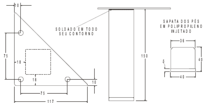
Fig 6 - Pé do armário (medidas em mm)
