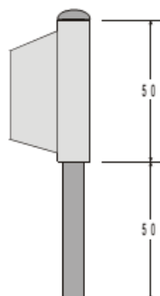
Fig 14 - Macho da dobradiça da porta (medidas em mm)
