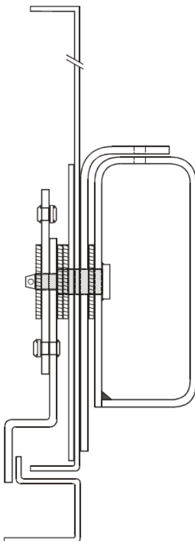
Fig 15 - Sistema de trancamento da porta montado
