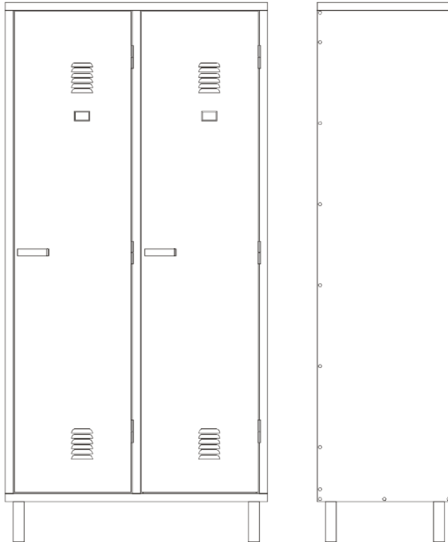
Fig 1 - Vista frontal e lateral do armário
