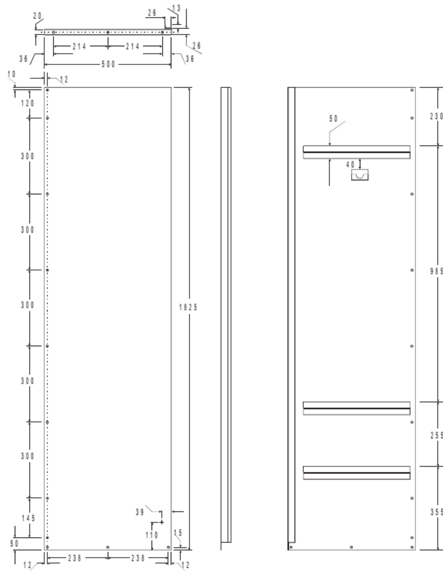
Fig 8 - Vista da lateral direita do armário (medidas em mm)
