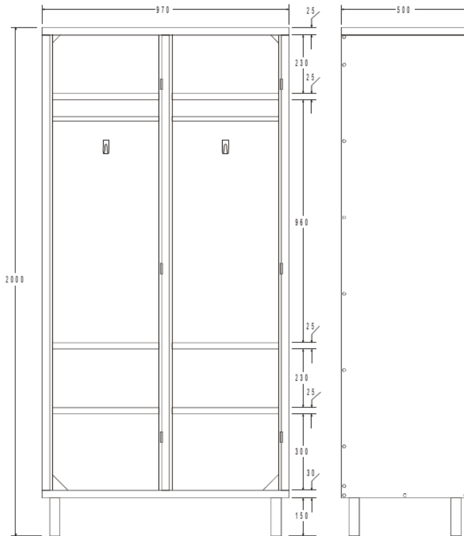
Fig 2 - Dimensões do armário (medidas em mm)
