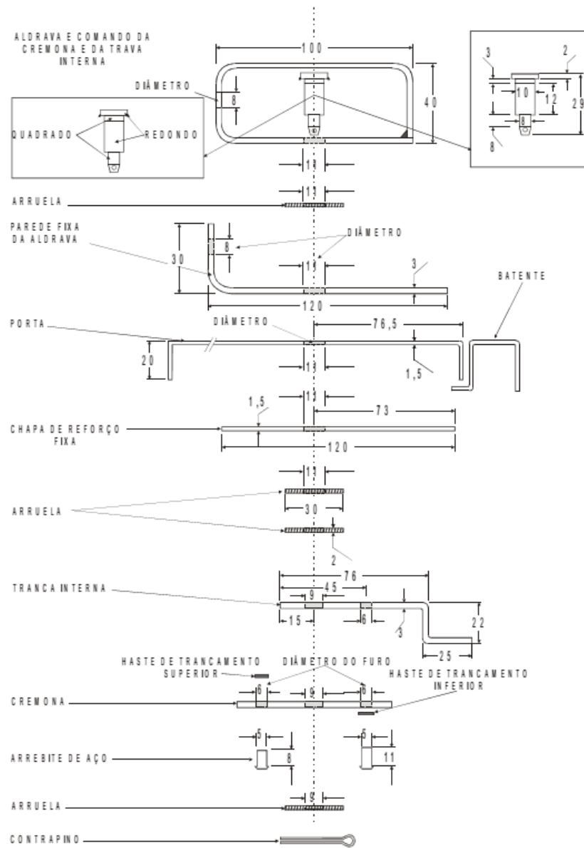
Fig 16 - Sistema de trancamento da porta desmontado (medidas em mm)
