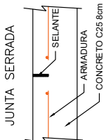
Detalhamento piso quadra Sem escala
