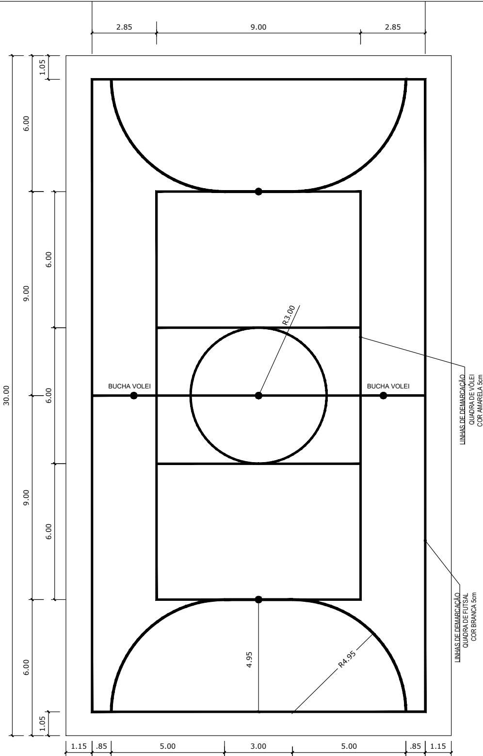
Planta baixa quadra Sem escala
