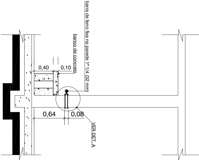
Corte detalhe barra de ferro fixa na parede
