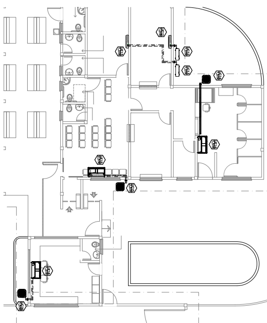
02 PLANTA BAIXA MÓDULO REVISTA-PORTARIA ESPERA EXTERNA ESCALA: 1:75
