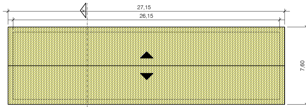
PLANTA DE COBERTURA Esc. 1/200
