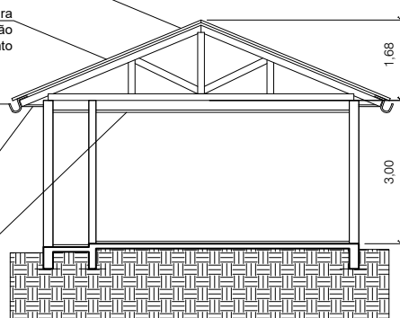
CORTE AA' Esc. 1/125
