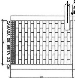
SUMIDOURO EM ALVENARIA TIPOLOS MACIO EM CRIVO TAMPA EM LAJE PREMOLDADA ESP. 13 CM
