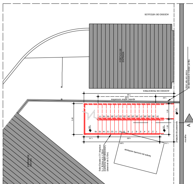
PROPOSTA 1 - PLANTA BAIXA - 1/50
