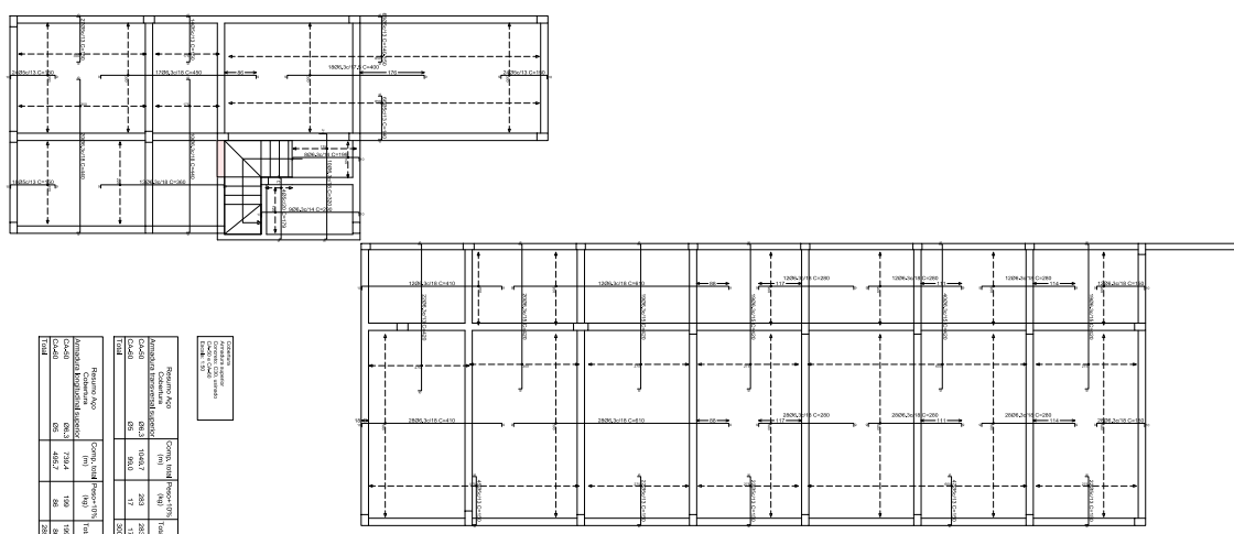
ARM. NEGATIVA LAJES - COBERTURA ESCALA: 1 / 50
