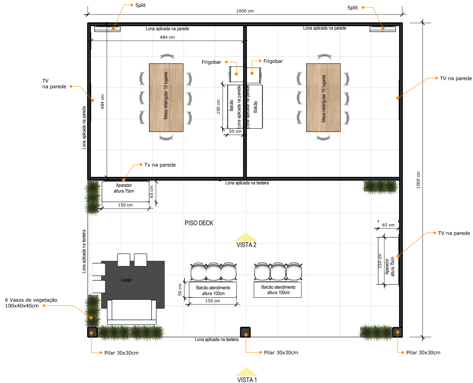
PLANTA BAIXA
