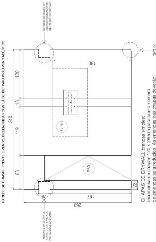
PLANTA DE CHAPAS DE DRYWALL - ESC.: 1/50
