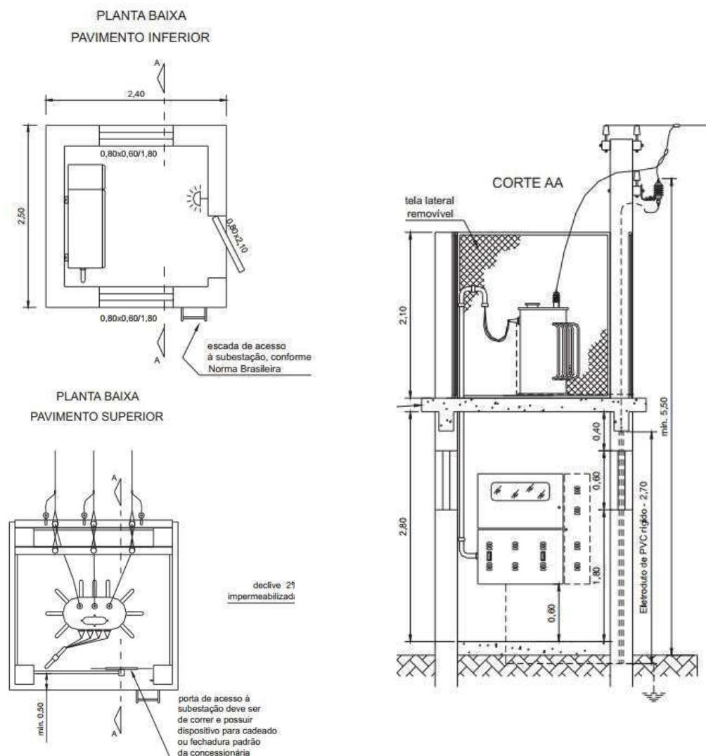
Figura 04- Planta baixa dos Pavimentos Inferior e Superior e Corte AA
