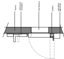
CORTE TRANSVERSAL CONJUNTO
