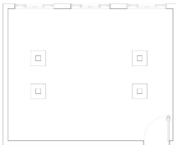
PLANTA SALA DE AULA EXEMPLO DE DISPOSIÇÃO DE ESCORAS
