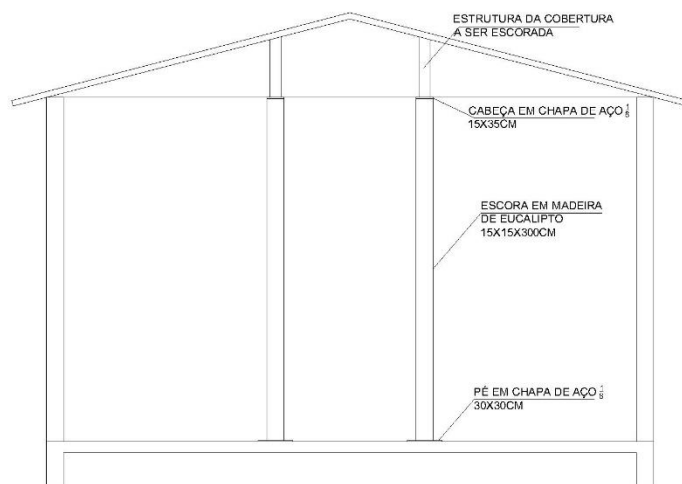
CORTE ESQUEMÁTICO SALA DE AULA
