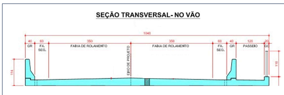
Fig. 5: Seção- tipo mínima exigida
