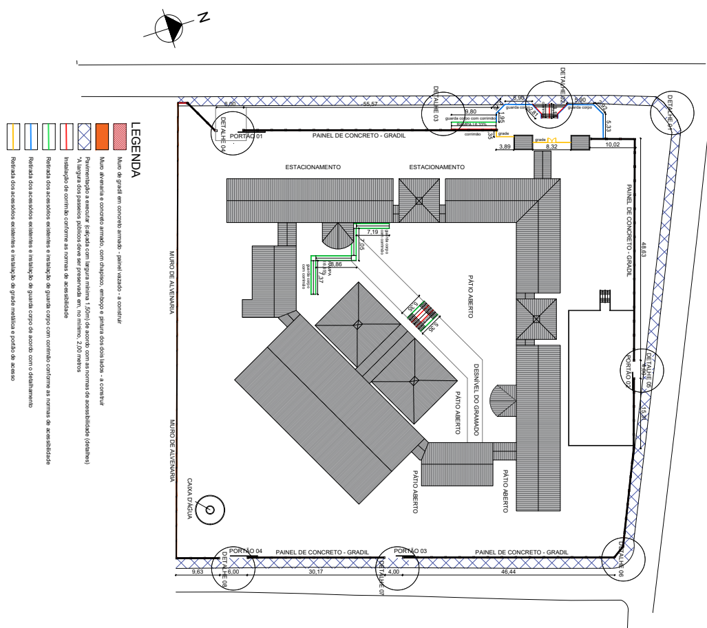
Planta de Localização e Cobertura Esc.: 1/250
