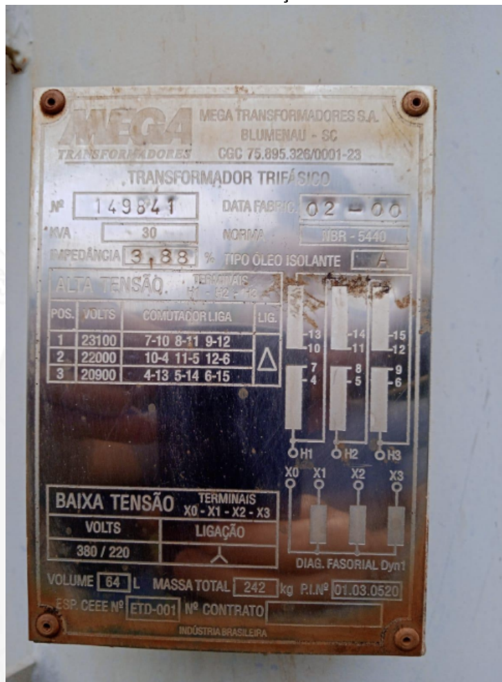
Foto 3: Placa com características do transformador
