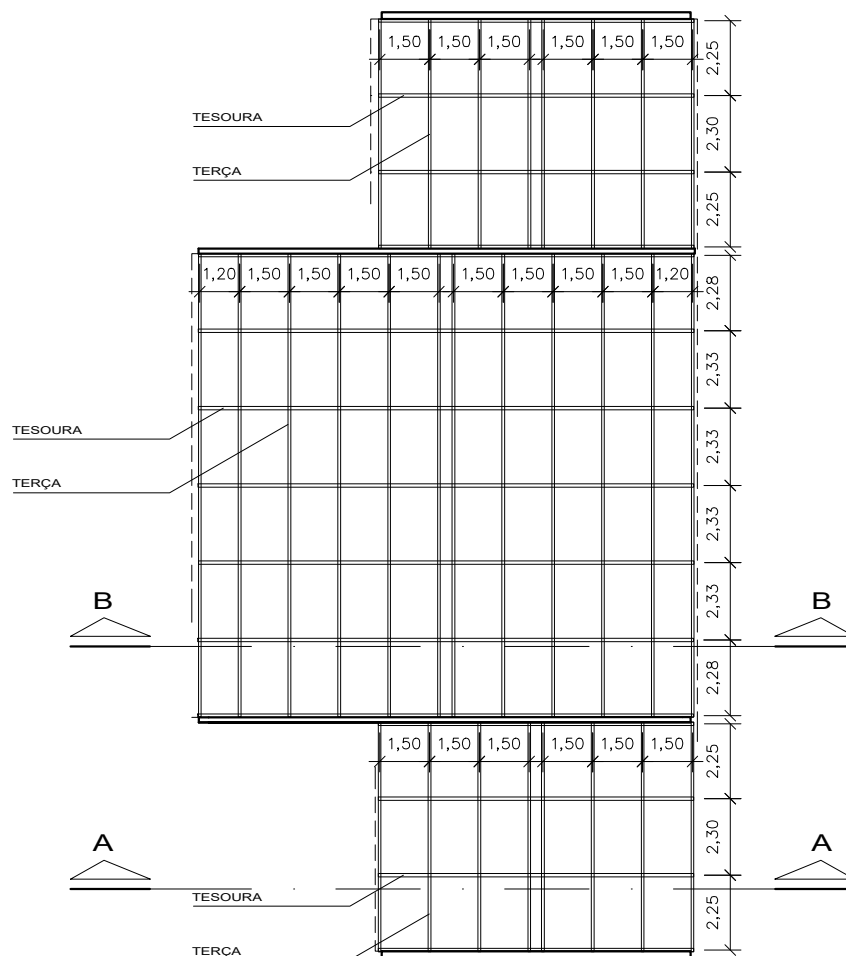
PLANTA DE COBERTURA - TRAMA BLOCO 03 E 04 A = 323,19 m² Esc.: 1/200
