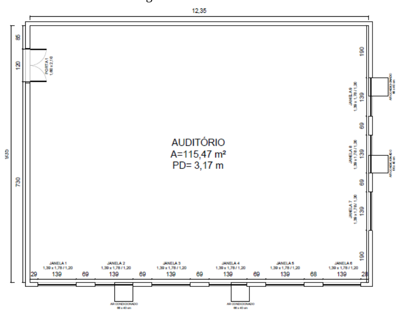
Imagem 2 - Croqui do Auditório - Sala 56
