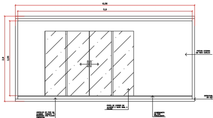
02 VISTA FRONTAL UN. 1/25
