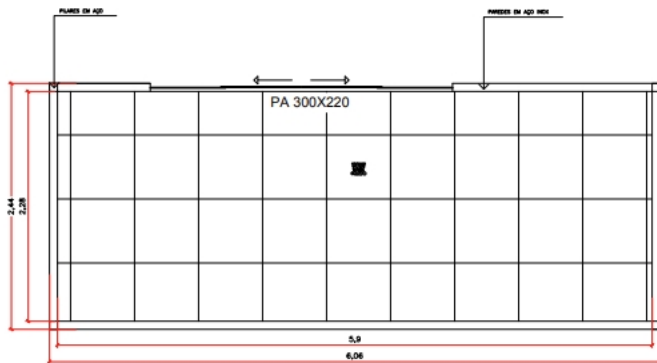
01 PLANTA BAIXA UN. 1/25
