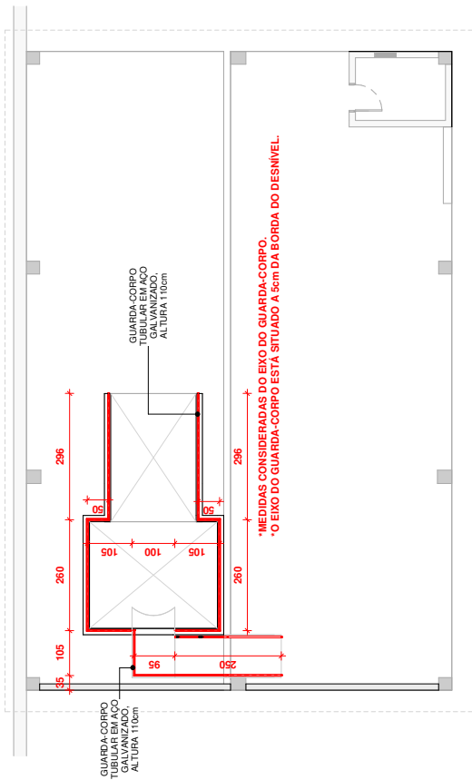
GUARDA-CORPO ARTEFATOS DE CIMENTO 1 : 100
