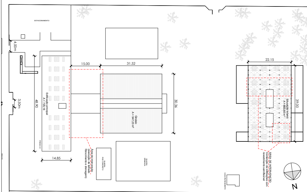
03 PLANTA BAIXA PARCIAL - DRENAGEM E.C.: 1/100
