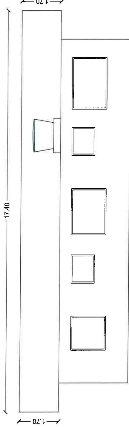
Fachada nordeste
