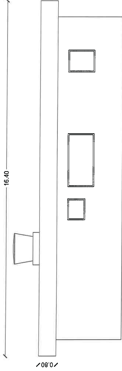
Fachada sudoeste
