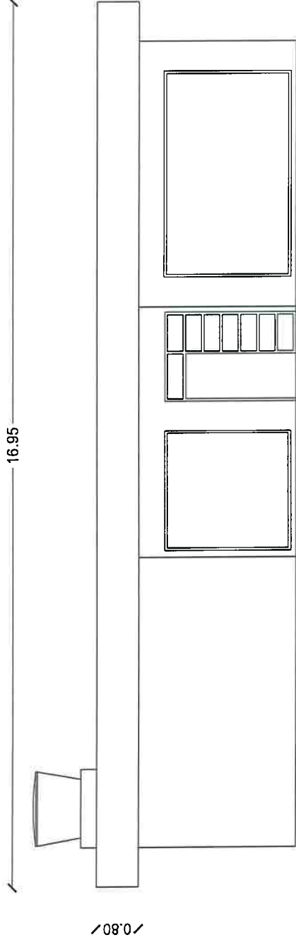
Fachada noroeste
