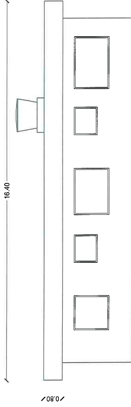
Fachada nordeste
