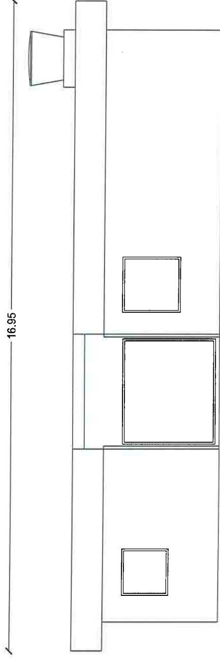
Fachada sudeste
