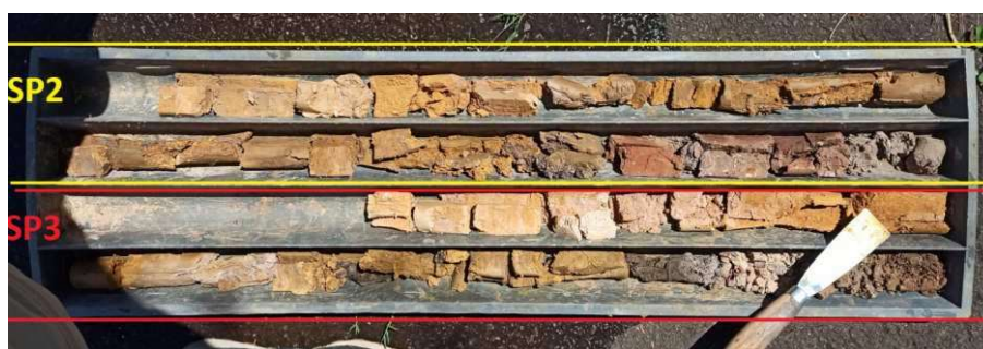
Figura 3 – Amostragem das Sondagens – Furos SP2 e SP3
