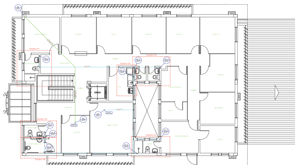
INSTALAÇÃO HIDRÁULICA - FUNDAMENTO SUPERIOR ESCALA: 1:50
