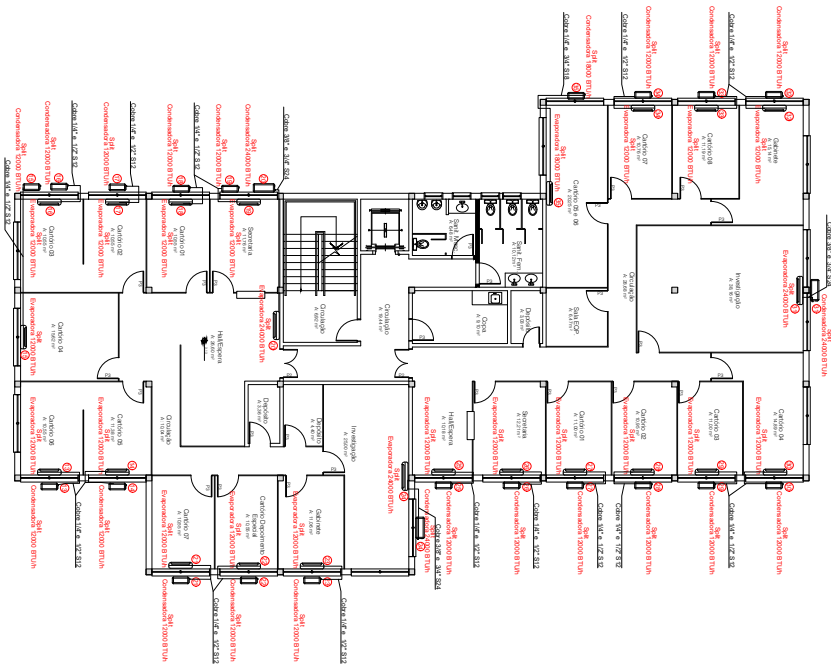
PLANTA BAIXA 2º PAVIMENTO - DEAM /DPPI Escala 1/50 Ass: SCS, Inc.
