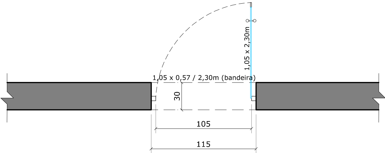
PLANTA BAIXA PORTA DE VIDRO ESC 1/25
