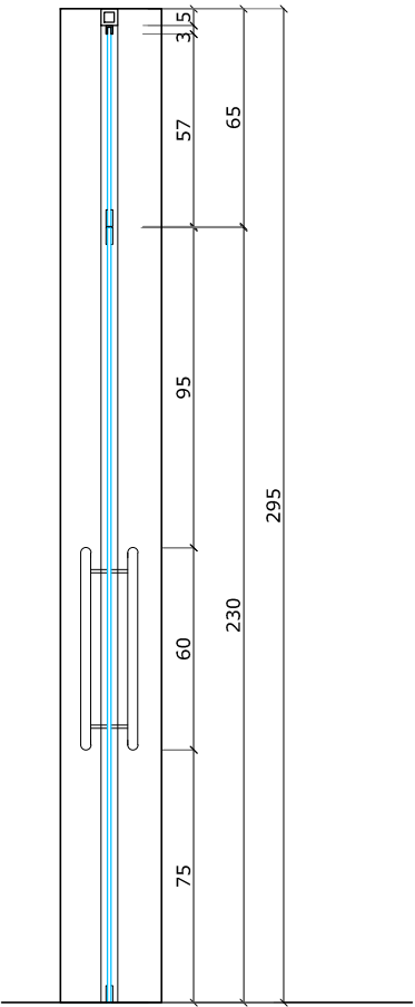
PERFIL PORTA DE VIDRO ESC 1/25
