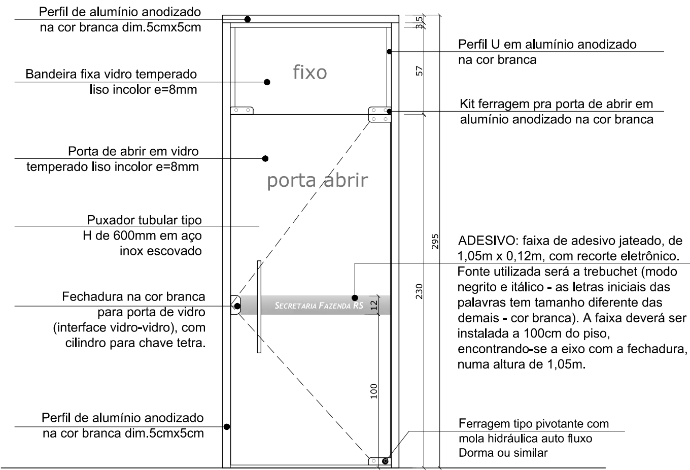
VISTA PORTA DE VIDRO ESC 1/25
