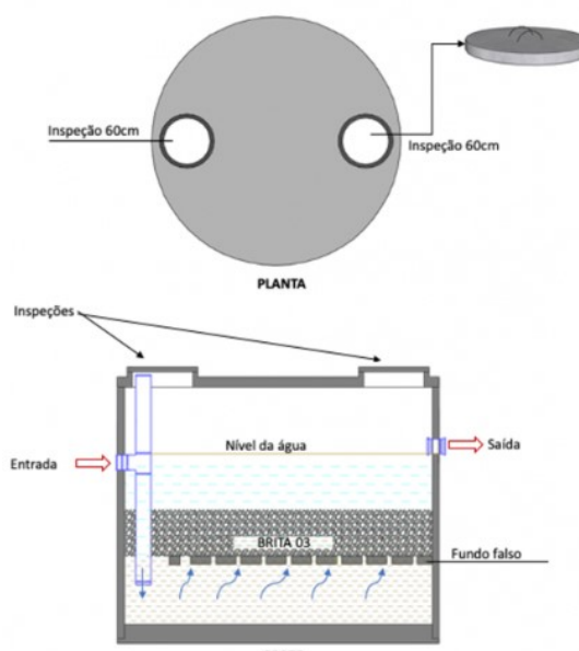
FILTRO ANAERÓBICO
