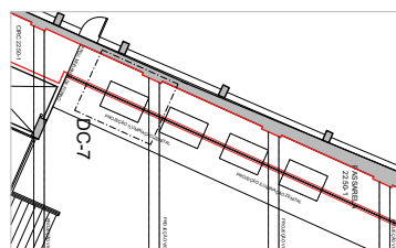
PLANTA BAIXA Escala 1/100 - NIVEL 22.50
